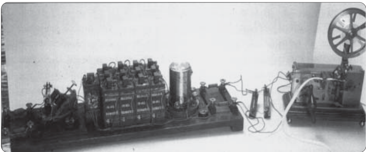
Ricevitore "Marconi" considerato il primo apparato militare della storia perché impiegato sulla corazzata "San Martino" nelle esperienze del 1897 tra l'Isola del Tino ed il Laboratorio Elettrico della Regia Marina a S. Bartolomeo. Con esso furono captati, per la prima volta, i segnali radio sino alla distanza record, per allora, di 18 chilometri dalla stazione trasmittente (Fondazione Marconi, collezione Maurizio Bigazzi, foto Cesare Gualdoni).
